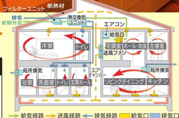
全館空調システムの概略図
