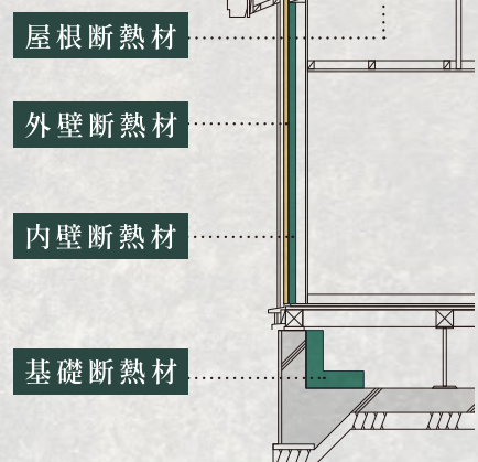
▲LEGANTIA (レガントシア) 断面図
