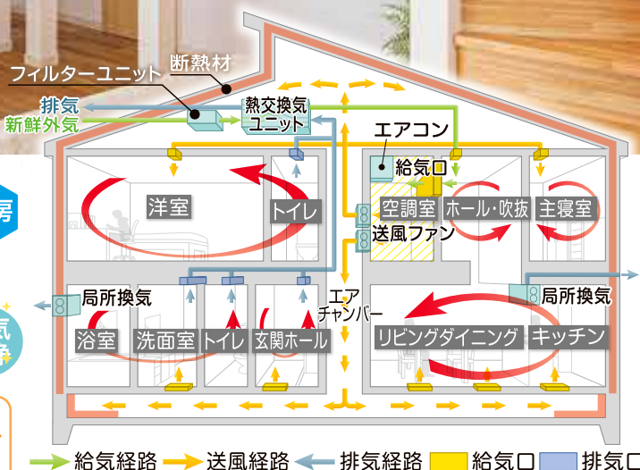
全館空調システムの概略図
