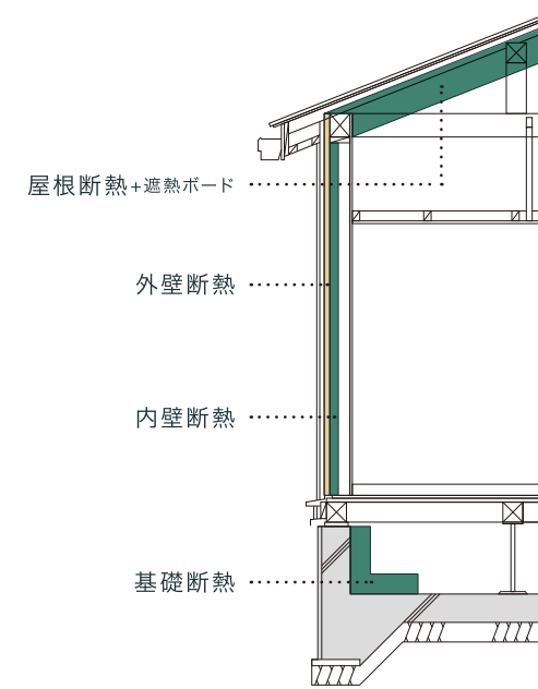
▲LEGANTIA（レガントシア）矩計図
