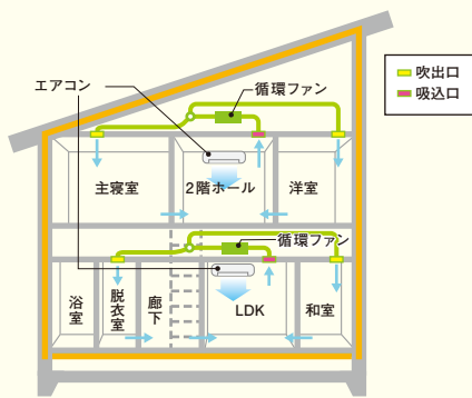
【Airフローシステムの空気の流れ】
