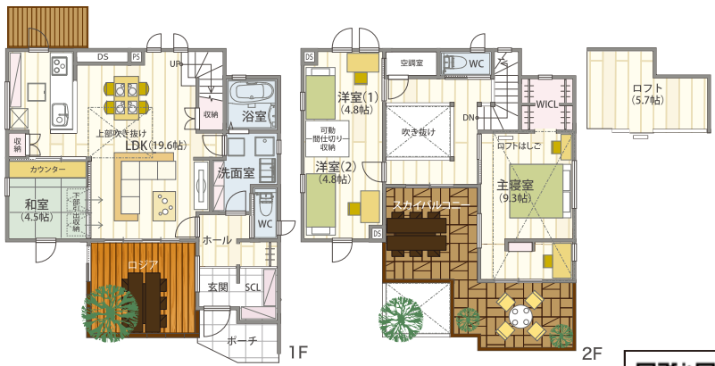
2階建34坪プラン
