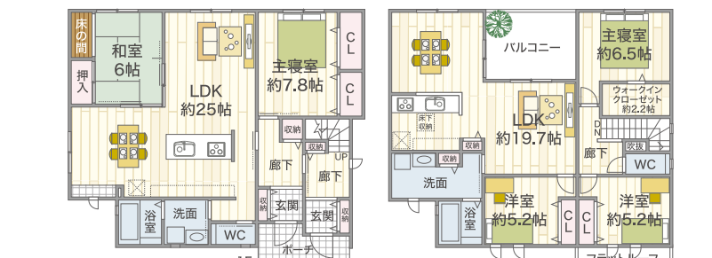
2階建54坪2世帯プラン
