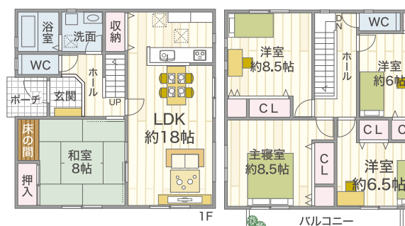
2階建39坪プラン
