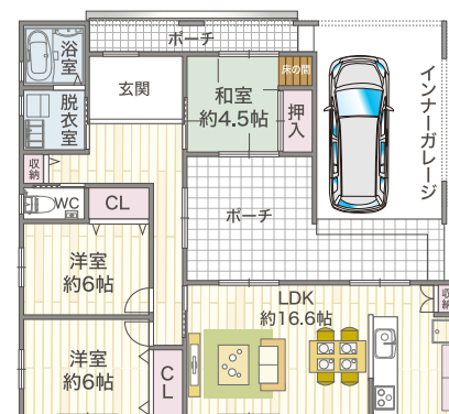
平屋25坪プラン
