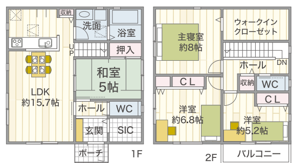
2階建32坪プラン
