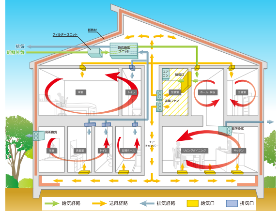
全館空調システムの概略図 (YUCACOシステム)
